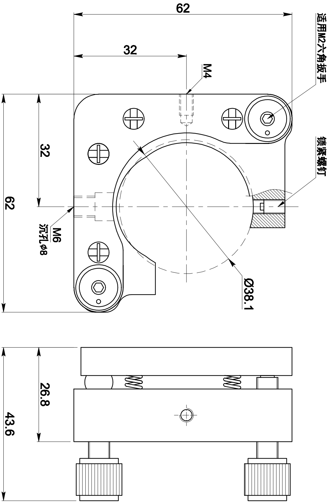
GCM-082316M 外形图
