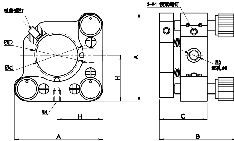
GCM-0828 系列外形图
