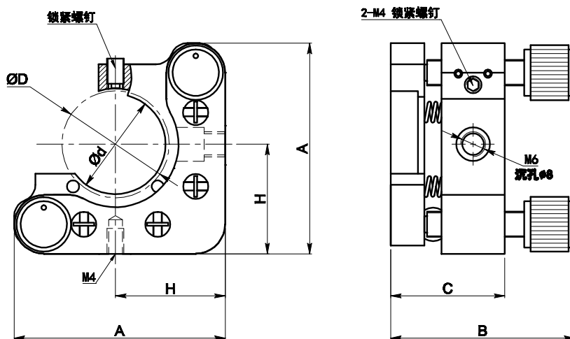
GCM-0818 系列外型图
